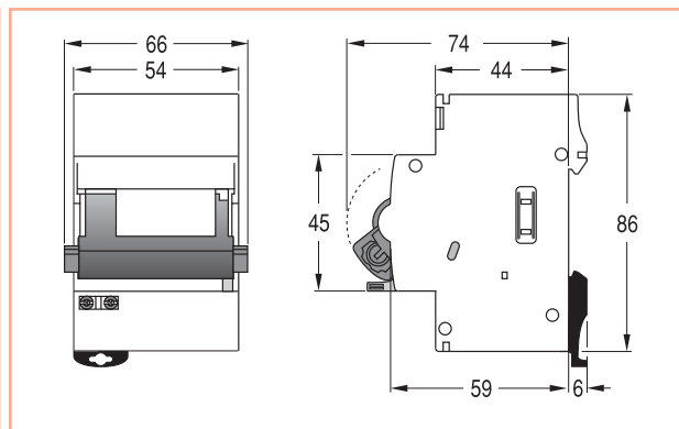
Моторный привод - Tele МР
